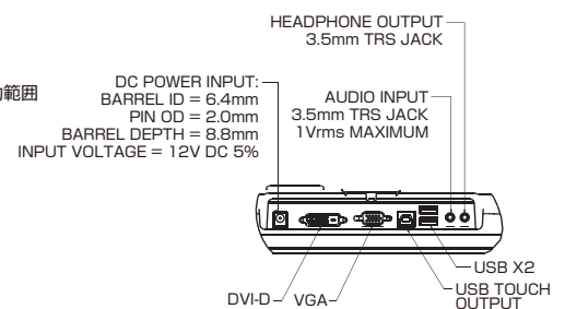
コネクタ部
