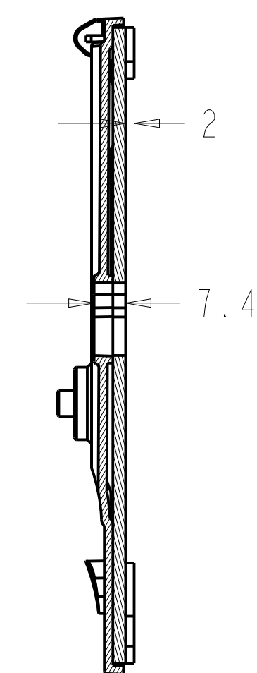
SECTION V-V
