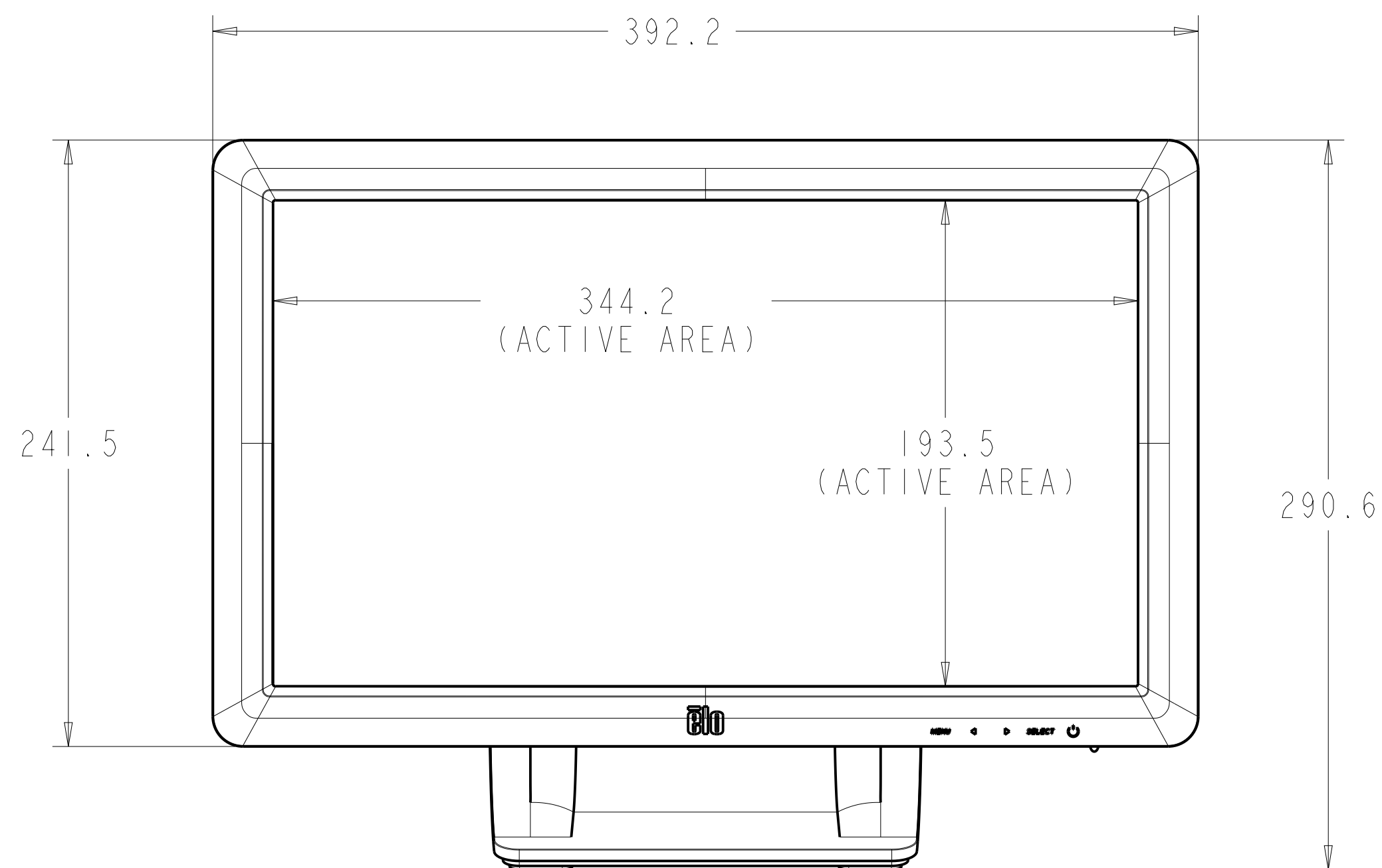
SCALE 0.5
