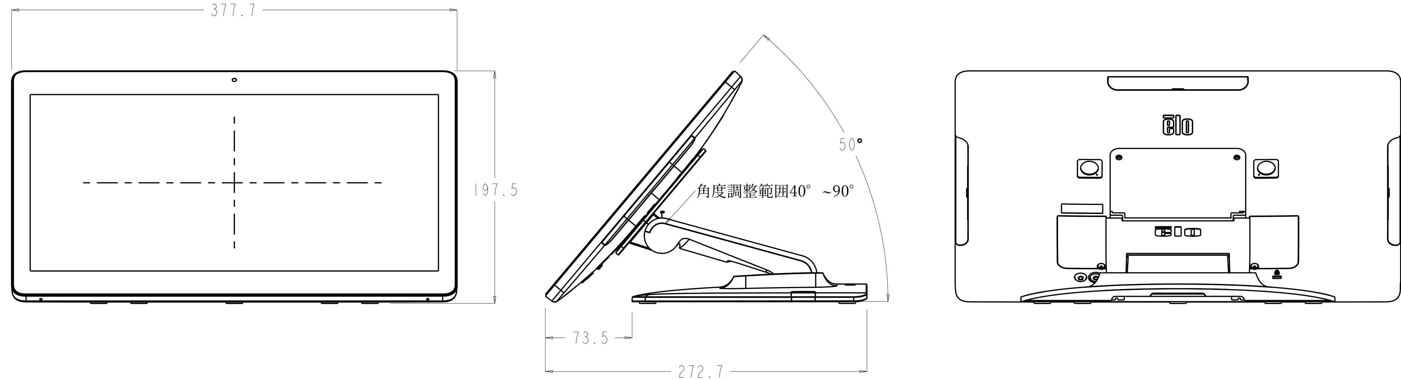
オプションスタンドE044162をLow Position40° で取り付けた場合
