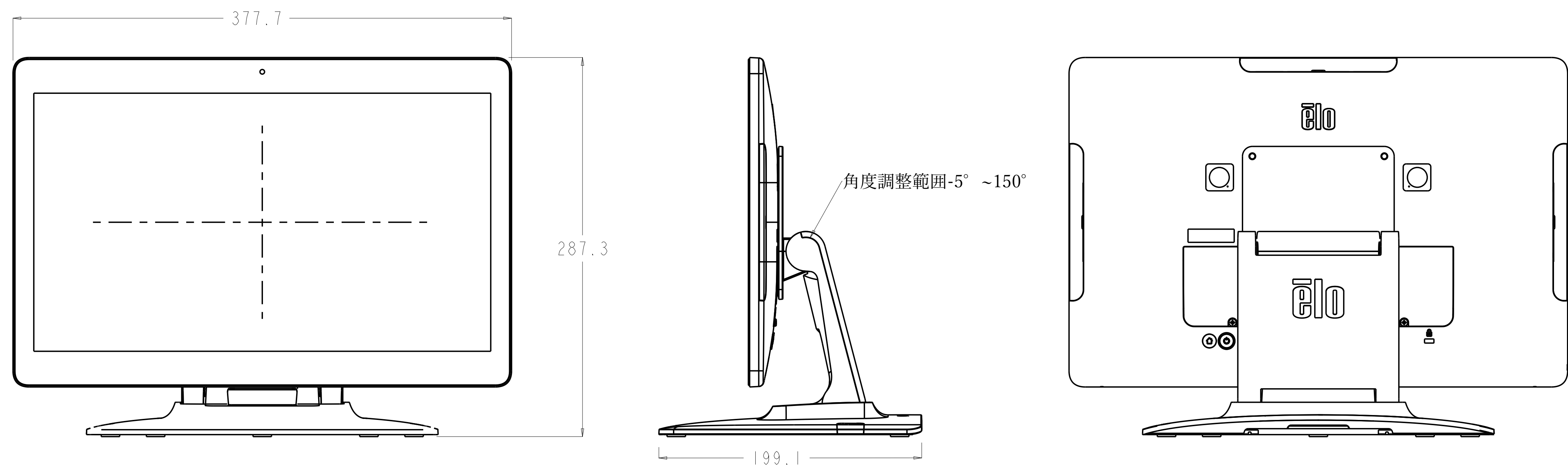
オプションスタンドE044162をHigh Position0° で取り付けた場合
