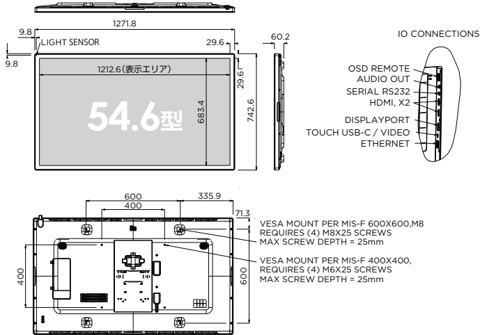
投影型静電容量方式モデル
