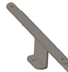
EMV Edge Bracket, 22 Android 4.0 (袋ラベル "22 A4") Qty. 1
