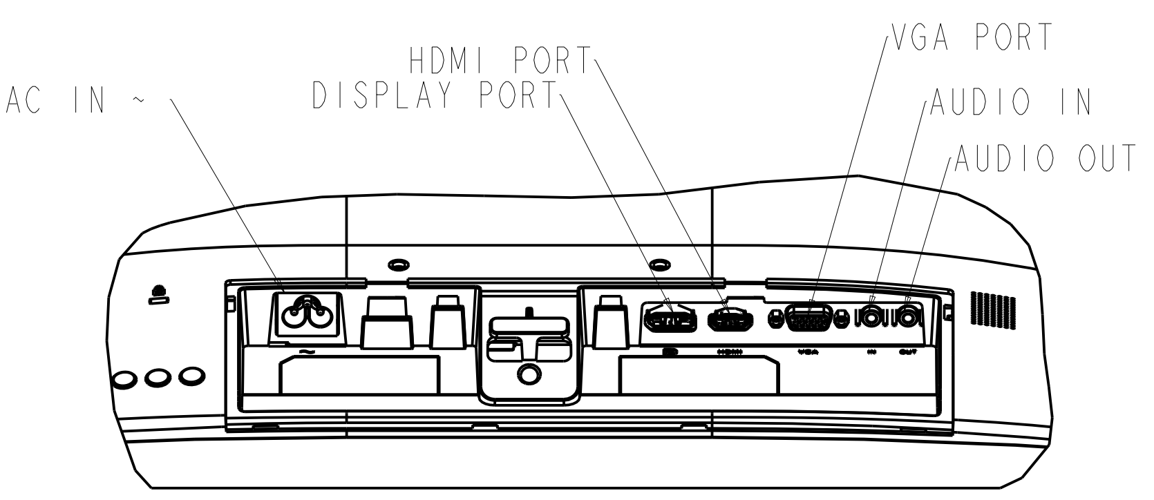
IO PANEL
