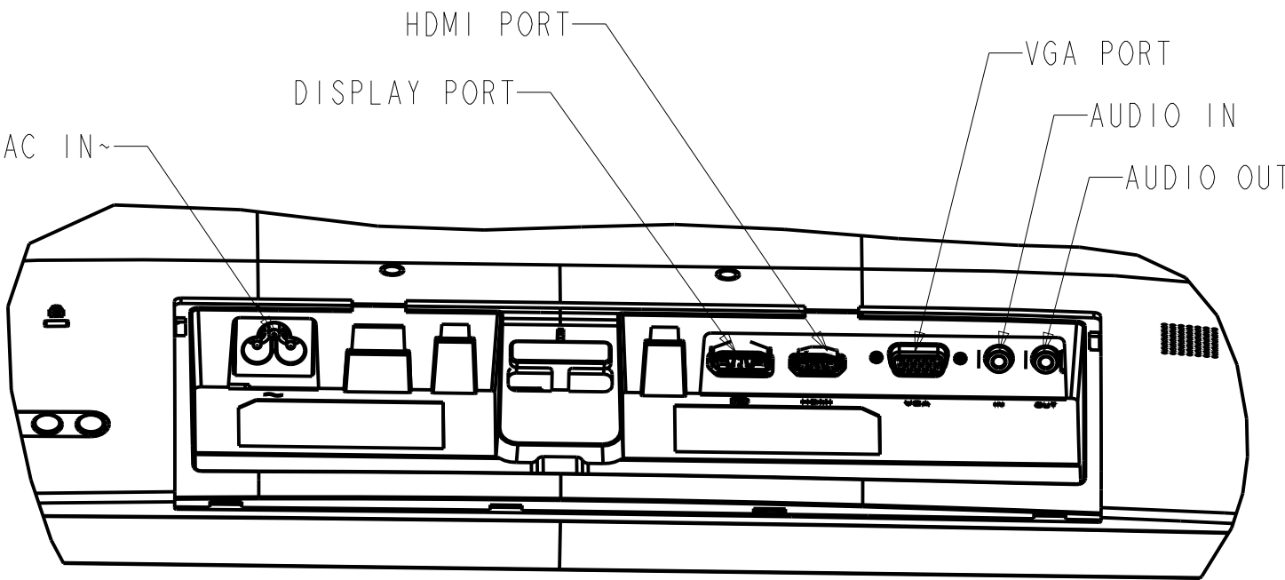
IO PANEL
