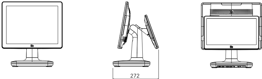
【オプションブラケット (E835969) を用いて背面にET1302Lを取り付けた場合】
