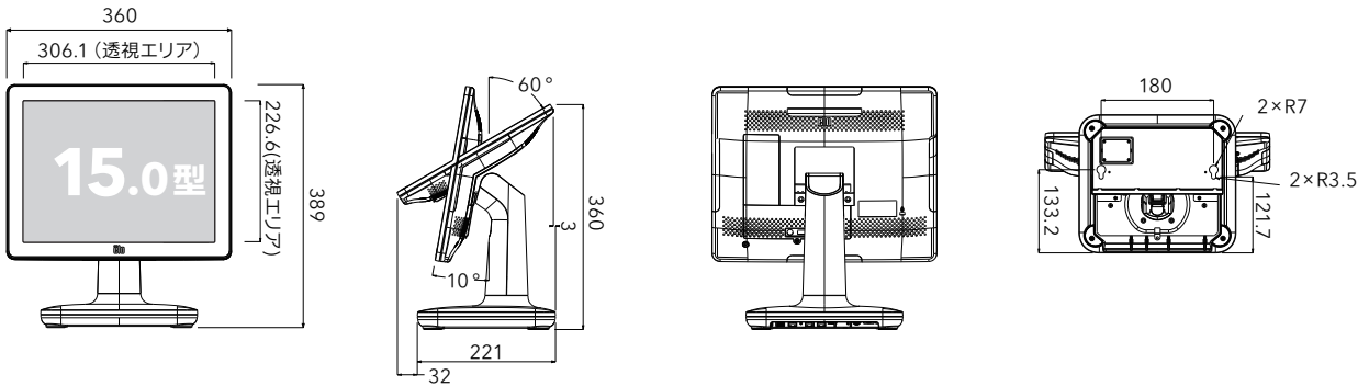
【オプションブラケット (E835969) を用いて背面にET1302Lを取り付けた場合】
